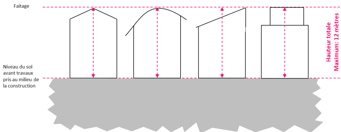
Hauteur maximale des constructions en zone Ns
