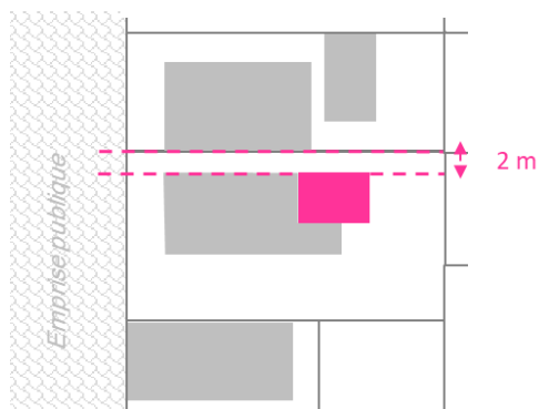
Implantation d'une extension à moins de 3m, mais dans le prolongement du bâtiment existant
