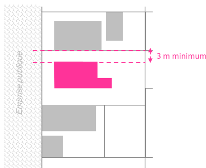
Implantation à minimum 3 mètres
