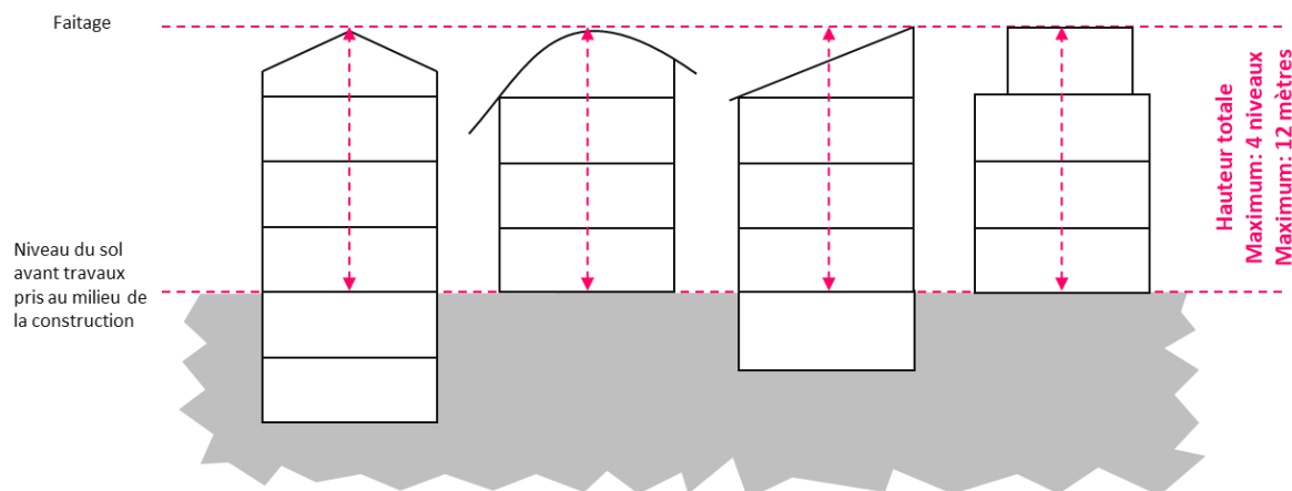
Hauteur maximale des constructions en zone Ua
