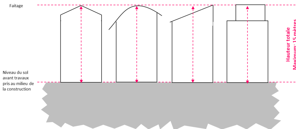
Hauteur maximale des constructions en zone A
