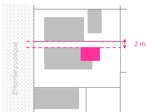
Implantation d'une extension à moins de 3m, mais dans le prolongement du bâtiment existant
