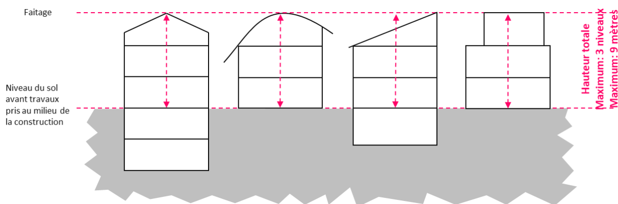
Hauteur maximale des constructions à usage de logement en zone Ux
