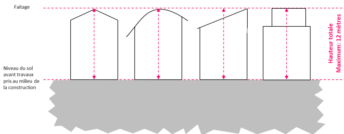
Hauteur maximale des constructions en zone Ax
