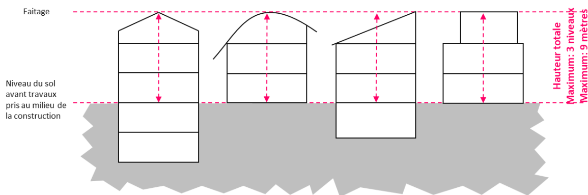
Hauteur maximale des constructions en zone Ah
