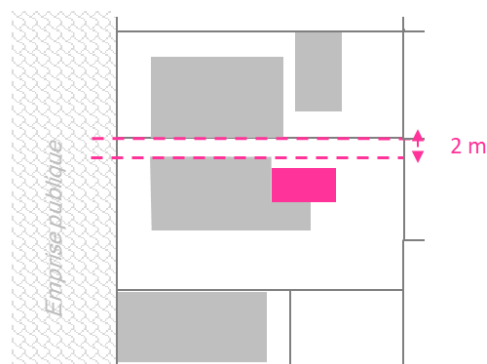
Implantation d'une extension à moins de 3m, mais avec un retrait supérieur par rapport au bâtiment existant
