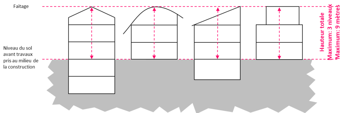
Hauteur maximale des constructions en zone Uc
