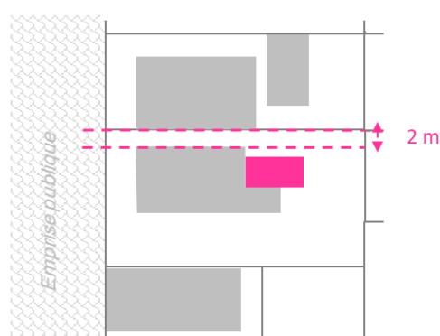
Implantation d'une extension à moins de 3m, mais avec un retrait supérieur par rapport au bâtiment existant
