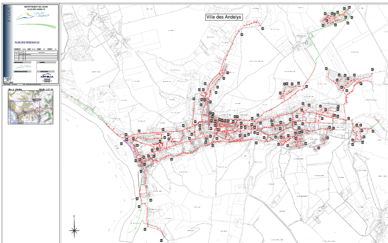
Schéma du réseau d'eaux usées de la commune des Andelys source : Schéma Directeur et diagnostic d'assainissement de Ville des Andelys, Artelia, septembre 2016
