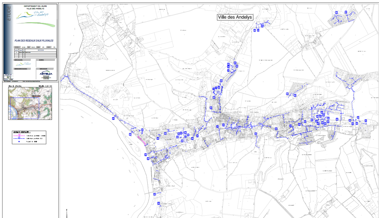
Schéma du réseau d'eaux pluviales de la commune des Andelys
